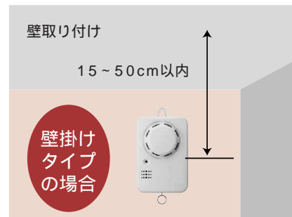
壁掛用火災警報器
