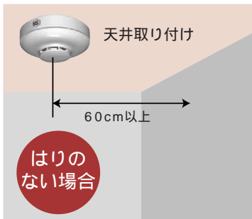
天井用火災警報器
