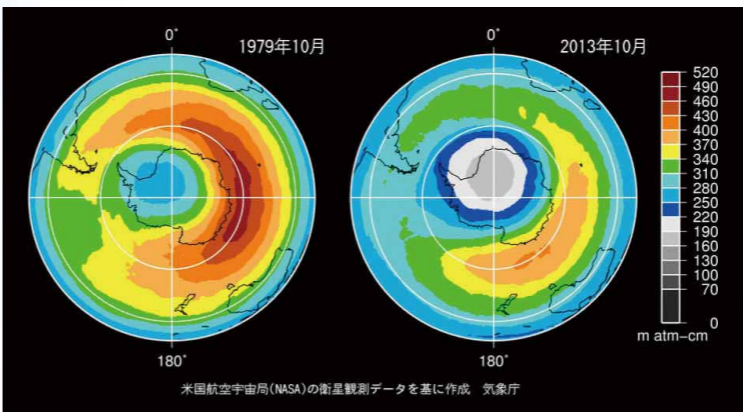
南極域のオゾンホールが現れる前の1979年と2013年それぞれの10月の平均オゾン全量の南半球分布。220m atm-cm以下の領域がオゾンホール。米航空宇宙局(NASA)提供の衛星データをもとに気象庁が作成。出典：気象庁ホームページより
